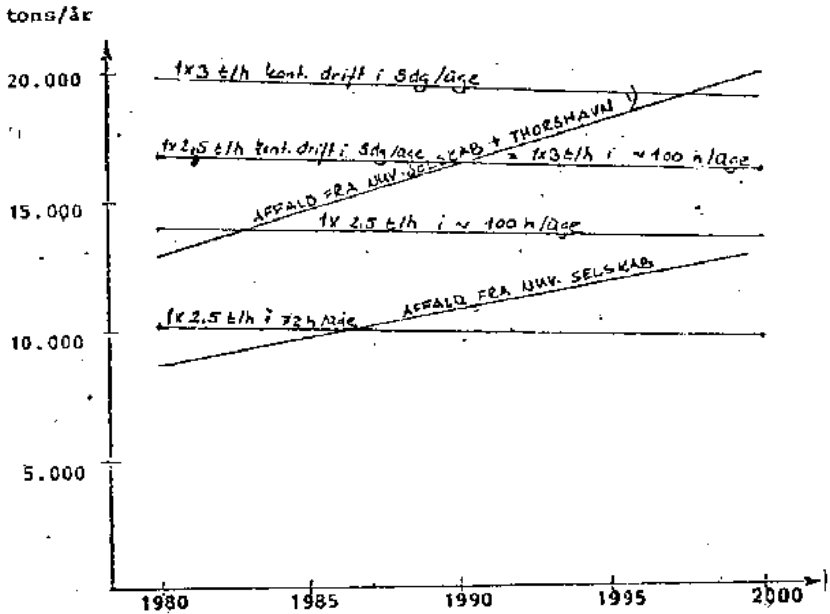
Fig. 1. Forbrændingsanlæggets kapacitet.
